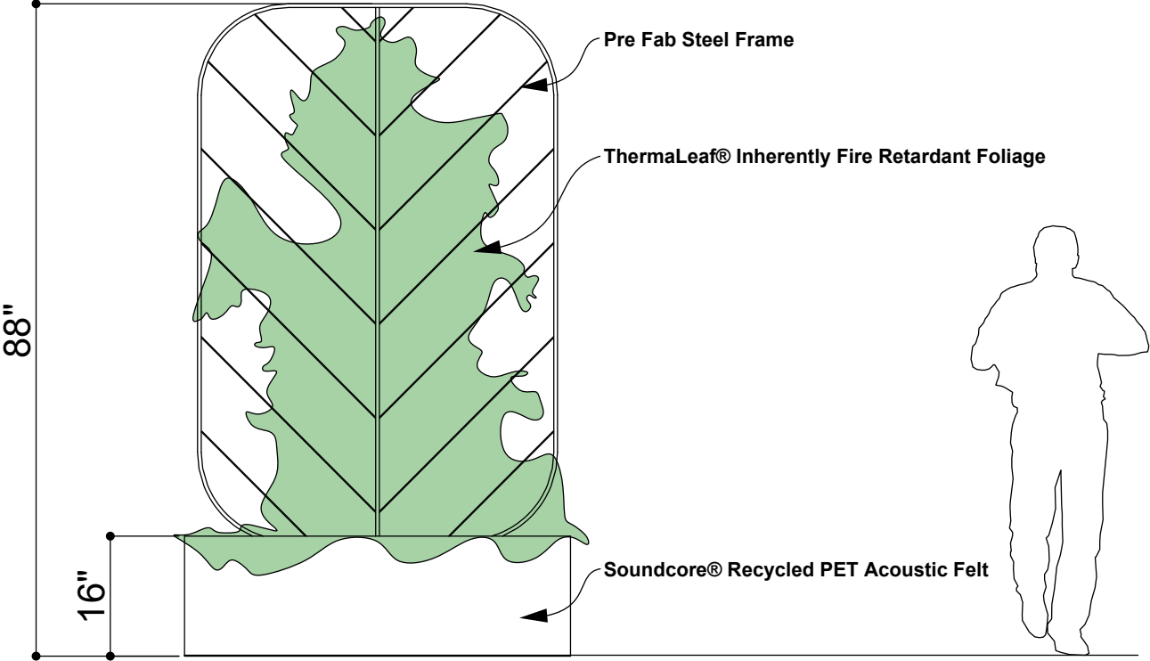
① ELEVATION 1
